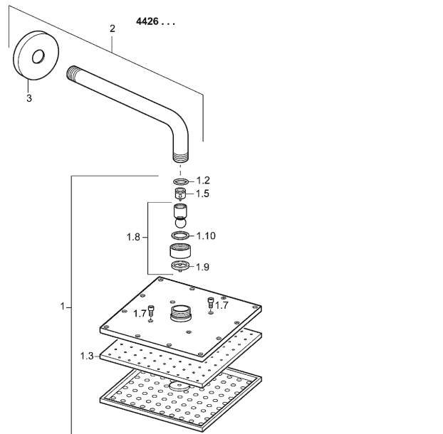
Producttekening
